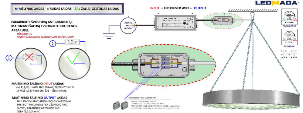
1. pav. Šviestuvo montavimas
