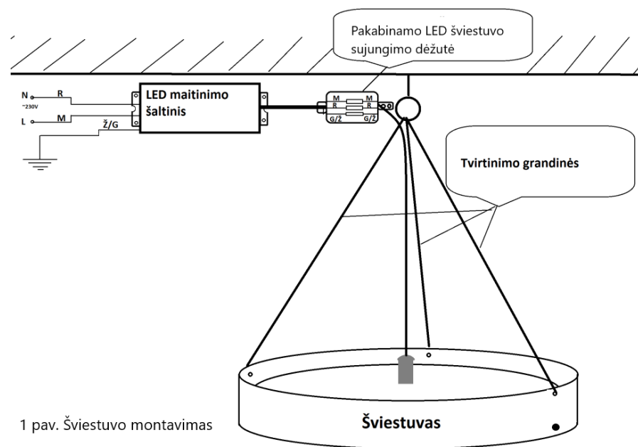
1. pav. Šviestuvo montavimas
