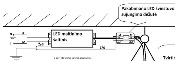
2 pav. Maitinimo šaltinio prijungimas
