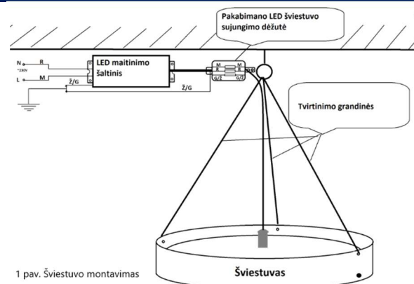
1 pav. Šviestuvo montavimas
