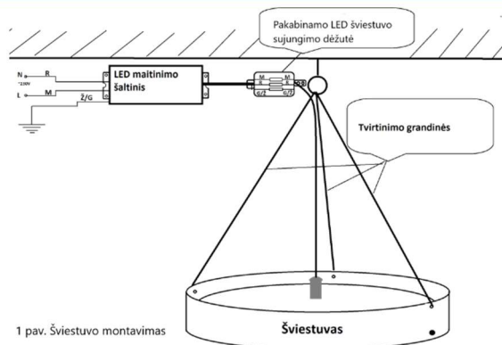
1 pav. Šviestuvo montavimas
