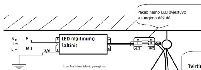
2 pav. Maitinimo šaltinio prijungimas
