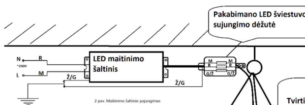
2 pav. Maitinimo šaltinio pajungimas
